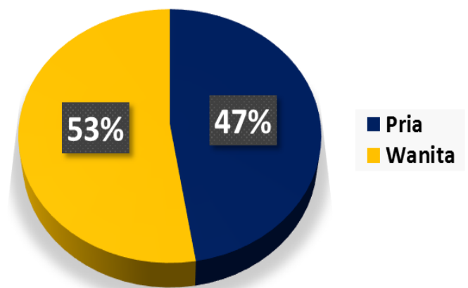
Gambar 3. Jenis Kelamin
