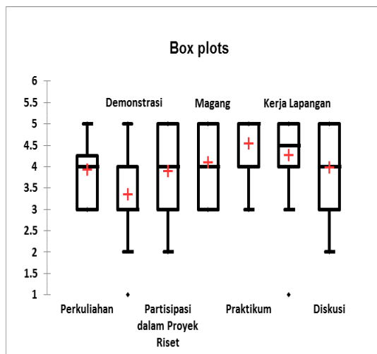
Gambar 7. Aspek Pembelajaran
